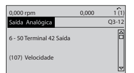
Ilustração 6.8 Passo 7: Utilize as teclas de navegação para cima/ para baixo para selecionar entre as diversas opções. Pressione [OK]
