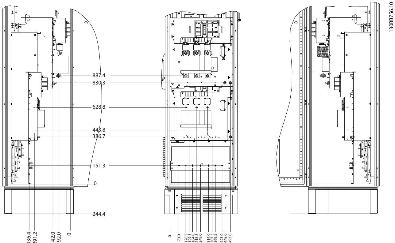
Ilustração 3.14 Terminal locations - Options Cabinet (Vistas esquerda, frontal e direita).
