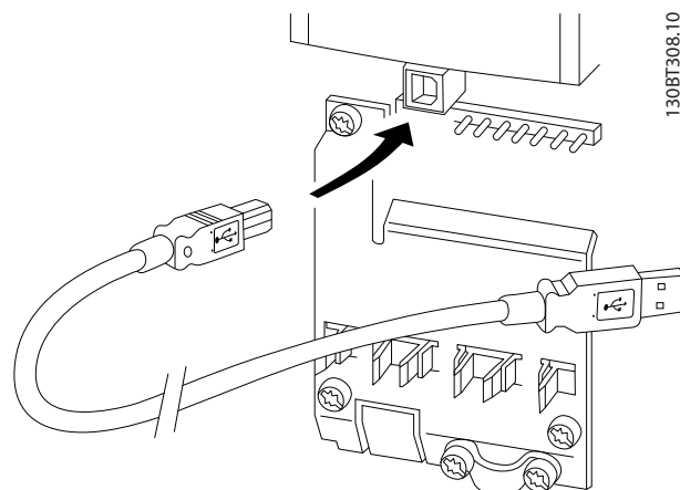
Ilustração 5.10 Para as conexões de cabo de controle, consulte a seção Terminais de Controle.
