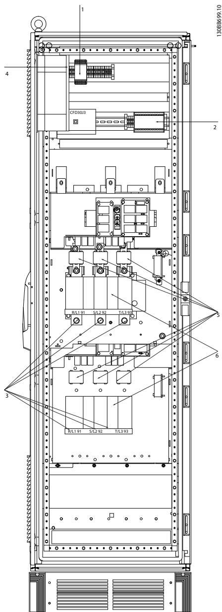
Ilustração 4.6 Gabinete para Opcionais, chassi de tamanho F9
