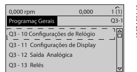
Ilustração 6.6 Passo 5: Utilize as teclas de navegação para cima/ para baixo, para rolar até Q3-12 Saídas Analógicas. Pressione [OK]
