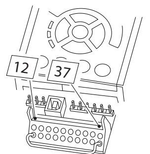
Ilustração 2.1 Coloque um jumper de conexão entre o terminal 37 e os 24 VCC.
