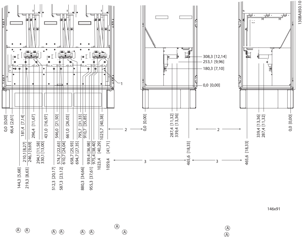
Ilustração 3.12 Localização dos terminais - Gabinete para Inversor (Visualização frontal, esquerda e direita). A placa da bucha está 42 mm abaixo do nível 0,0.
