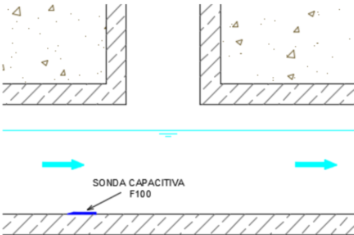
Ejemplo de instalación de la sonda F100 en el fondo de un canal de alivio
