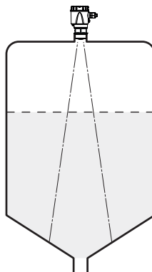
Fig. 10: Montagem do sensor de radar em reservatórios com fundo cônico
