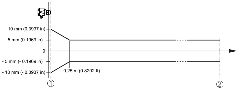
Fig. 6: Diferença de medição sob condições de referência 1)
