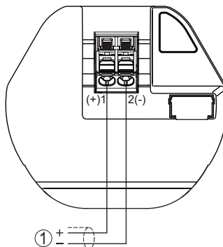
Fig. 19: Compartimento de conexões NivoRadar 7100
