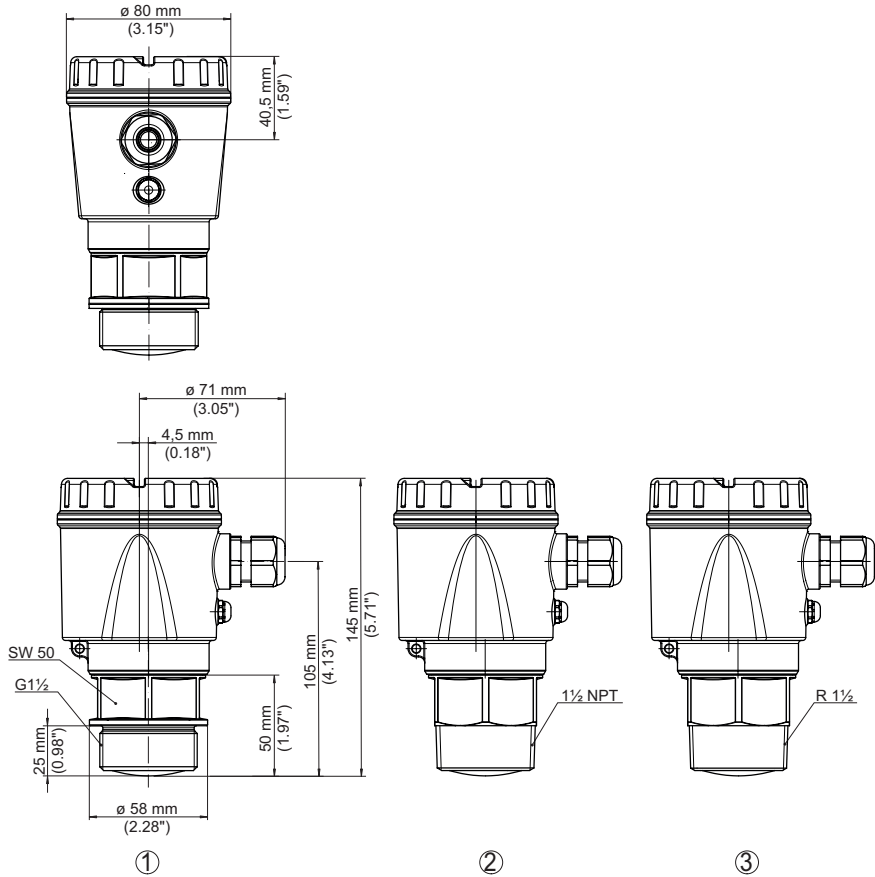
Fig. 7: Dimensões NivoRadar 7100
