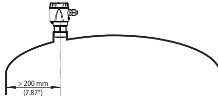
Fig. 9: Montagem do sensor de radar em teto de reservatório redondo
