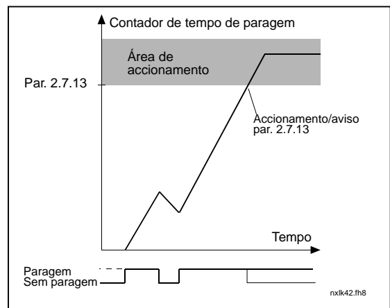
Figura 1- 21. Contagem do tempo de paragem
