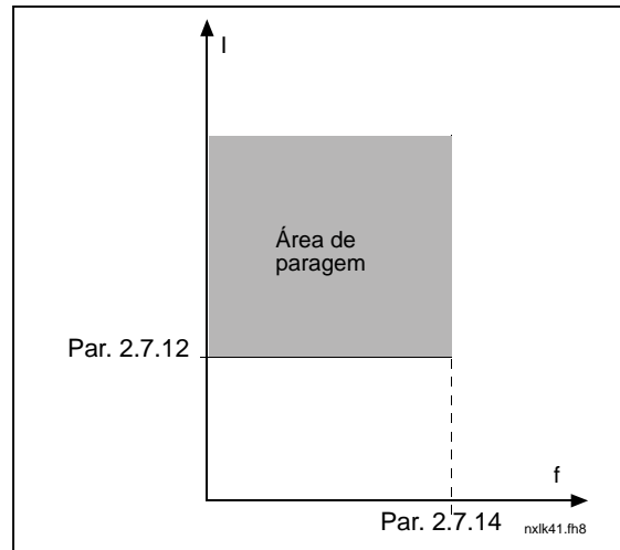
Figura 1-20. Definições de características de paragem
