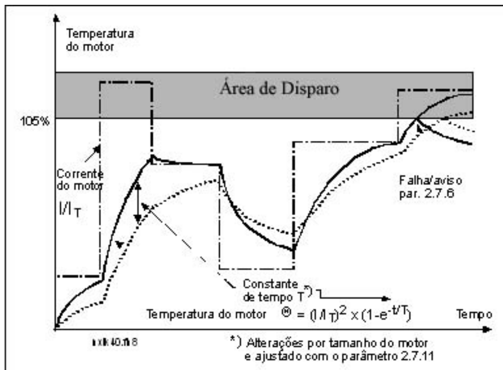
Figura 1- 19. Cálculo da temperatura do motor
