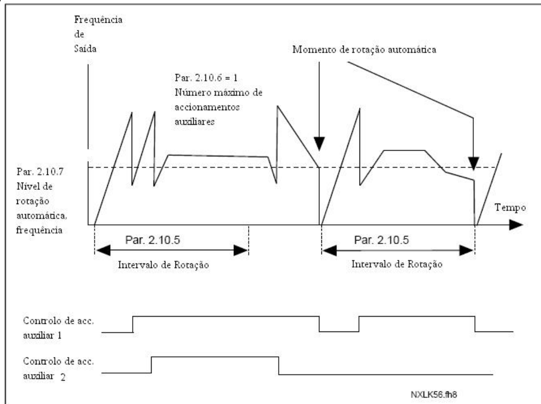
Figura 1-37. Intervalo e limites de comutação automática
