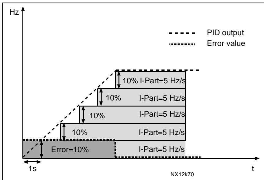
Figura 1-25. Funcionamento do controlador PID como um controlador I
