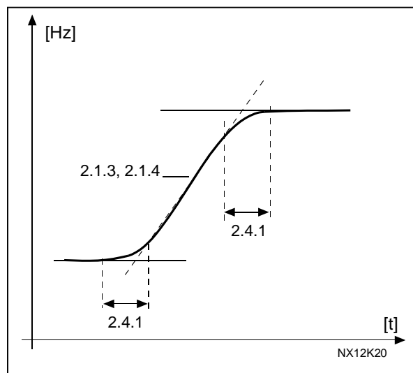
Figura 1-10. Aceleração/desaceleração (curva S)
