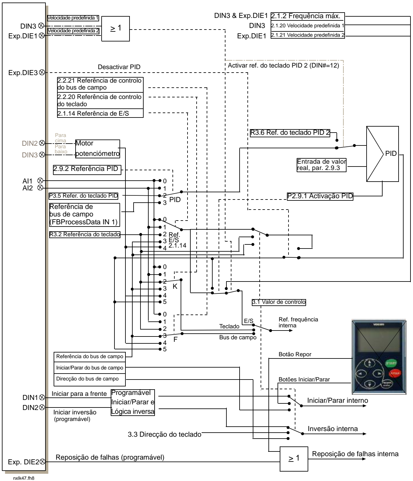
Figura 1-38. Lógica de sinais de controlo da Aplicação de Multi-Propósito
