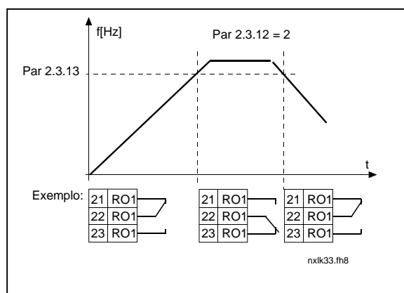
Figura 1-8. Supervisão da frequência de saída
