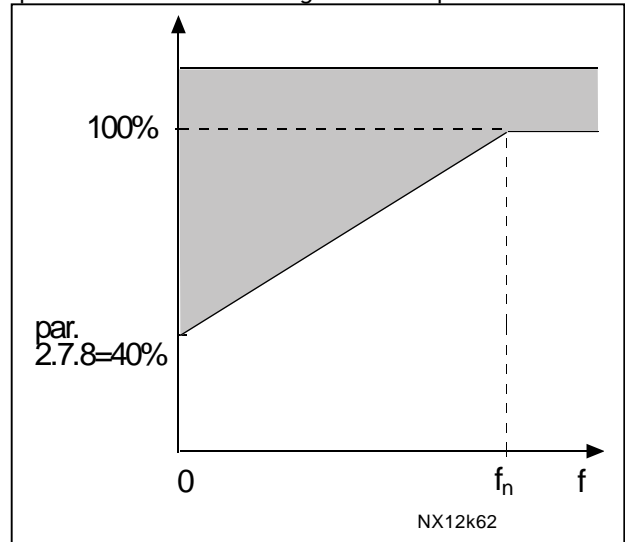
Figura 1- 18. Potência de refrigeração do motor
