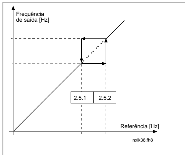
Figura 1- 14. Definição da área de frequência proibida
