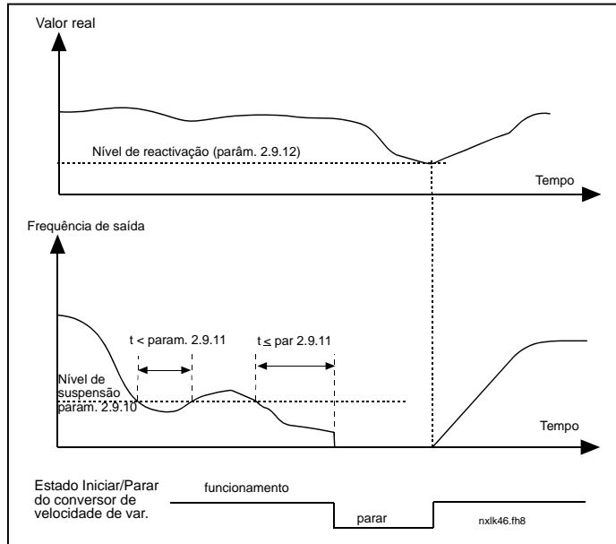
Figura 1- 29. Função adormecer do do conversor de frequência
