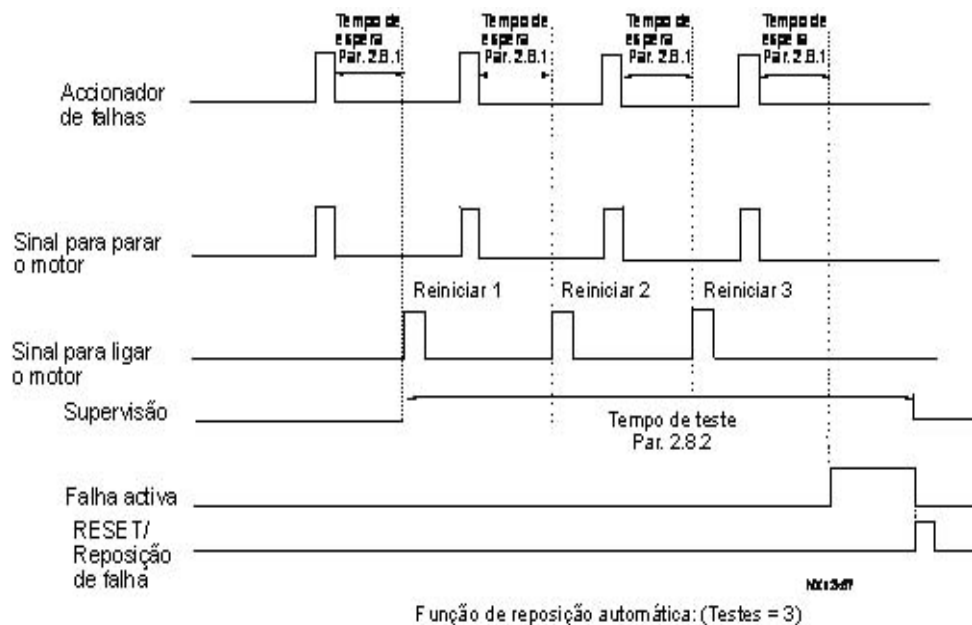
Figura 1-24. Rearranque automático.
