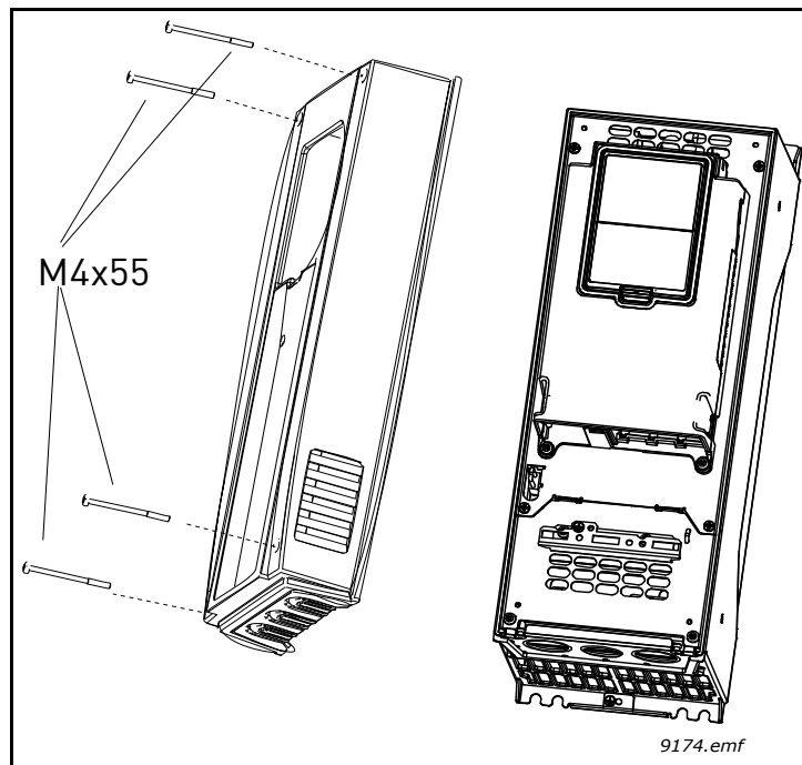
Figura 56. Abrir a tampa principal
