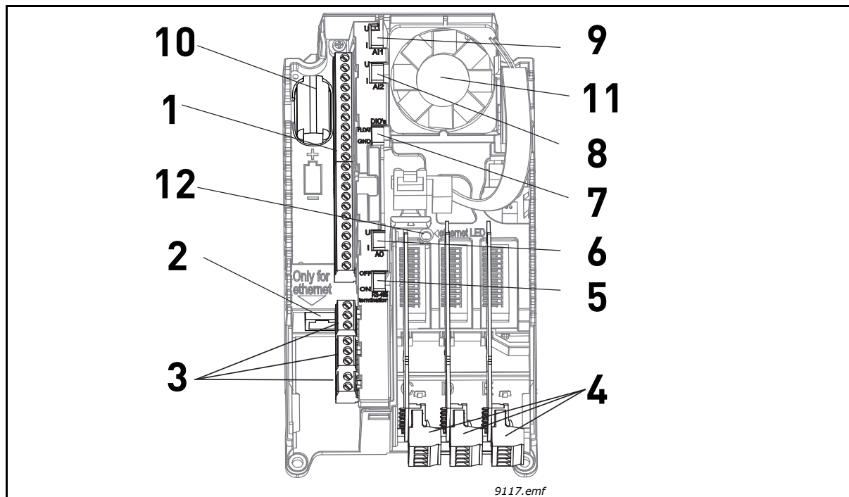
Figura 48. Localização dos componentes da unidade de controlo
