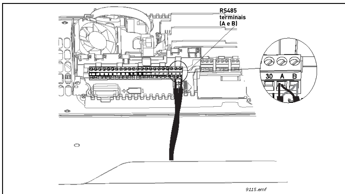
Figura 55. Ligar o cabo RS485
