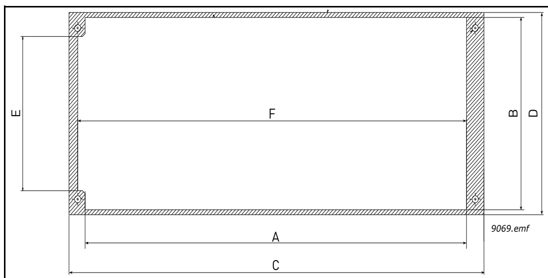
Figura 13. Dimensões do recorte para montagem com flange do MR4 ao MR6
