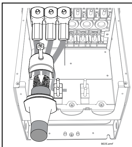
Figura 44. Expor as blindagens dos cabos
