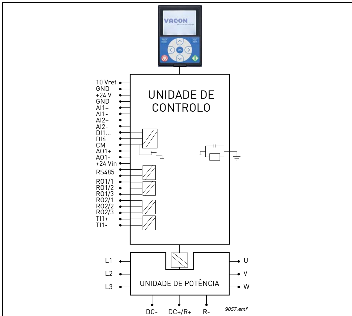
Figura 57. Barreiras galvânicas de isolamento
