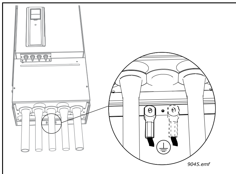
Figura 47. Ligar o condutor de protecção
