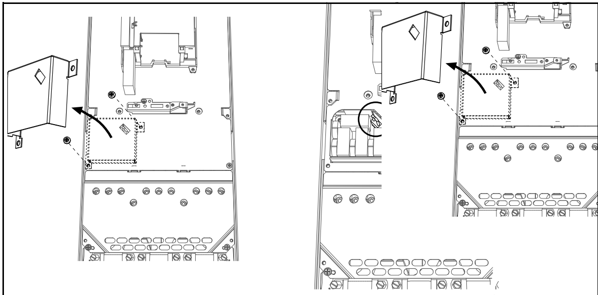
Figura 61. Retirar o jumper de EMC, MR7-8
