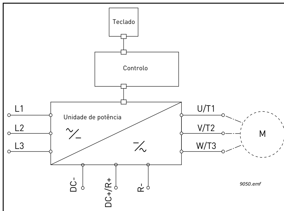
Figura 20. Esquema das ligações principais
