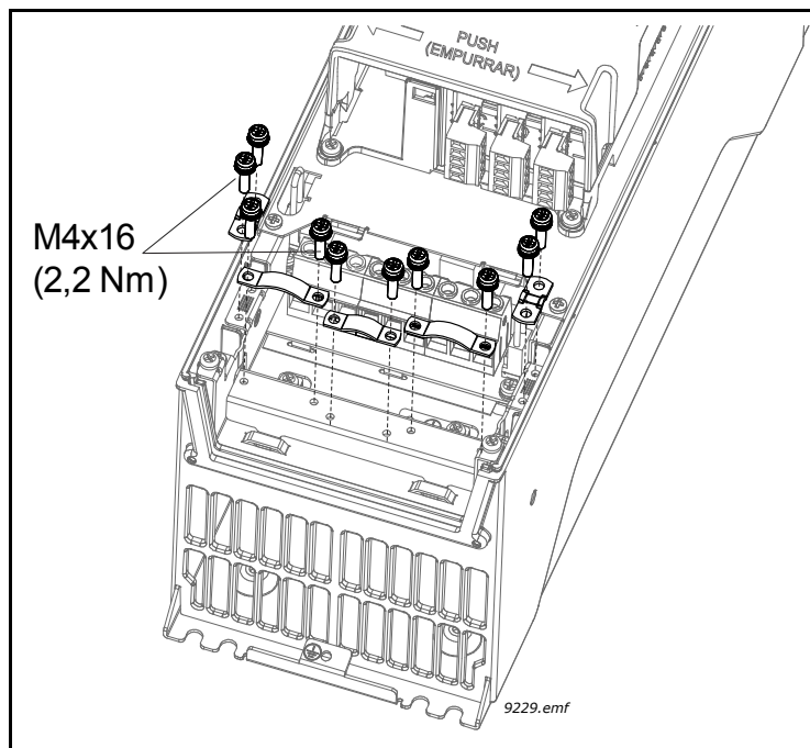
Figura 27. Soltar as braçadeiras para cabos
