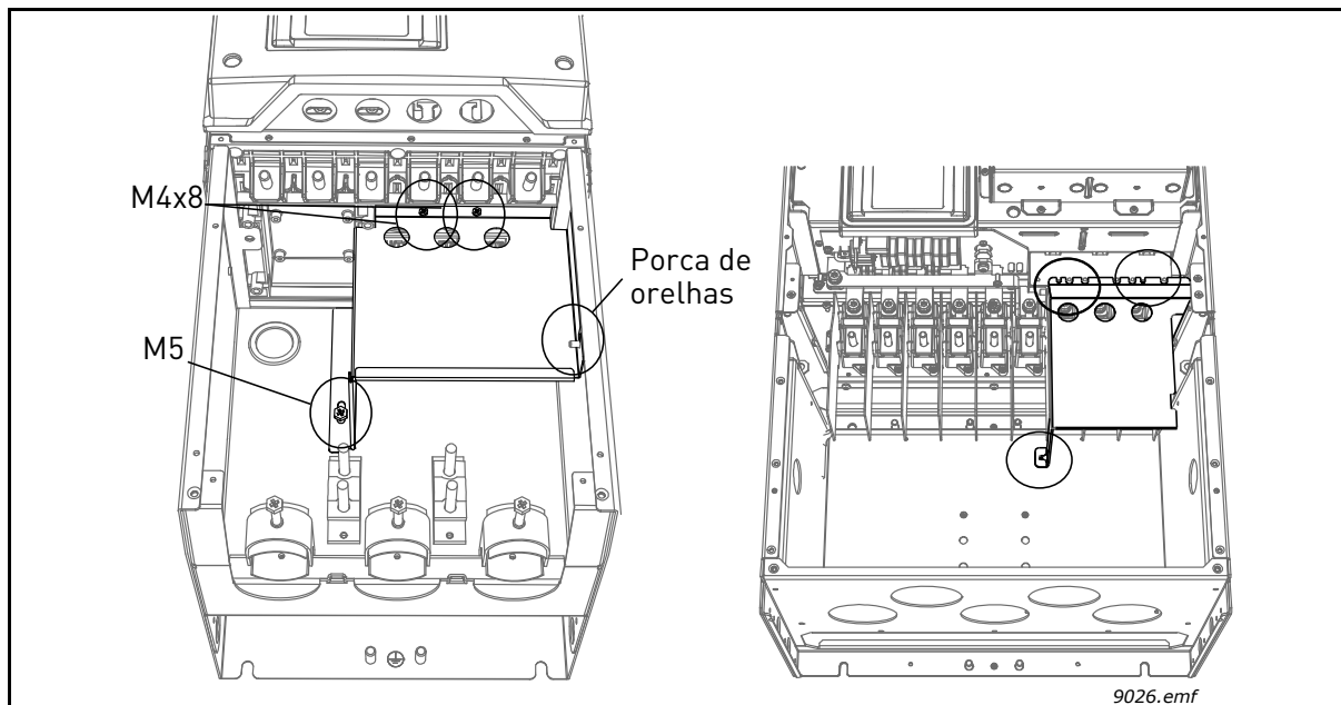
Figura 37. Retirar a placa de blindagem EMC, esquerda: MR8, direita: MR9
