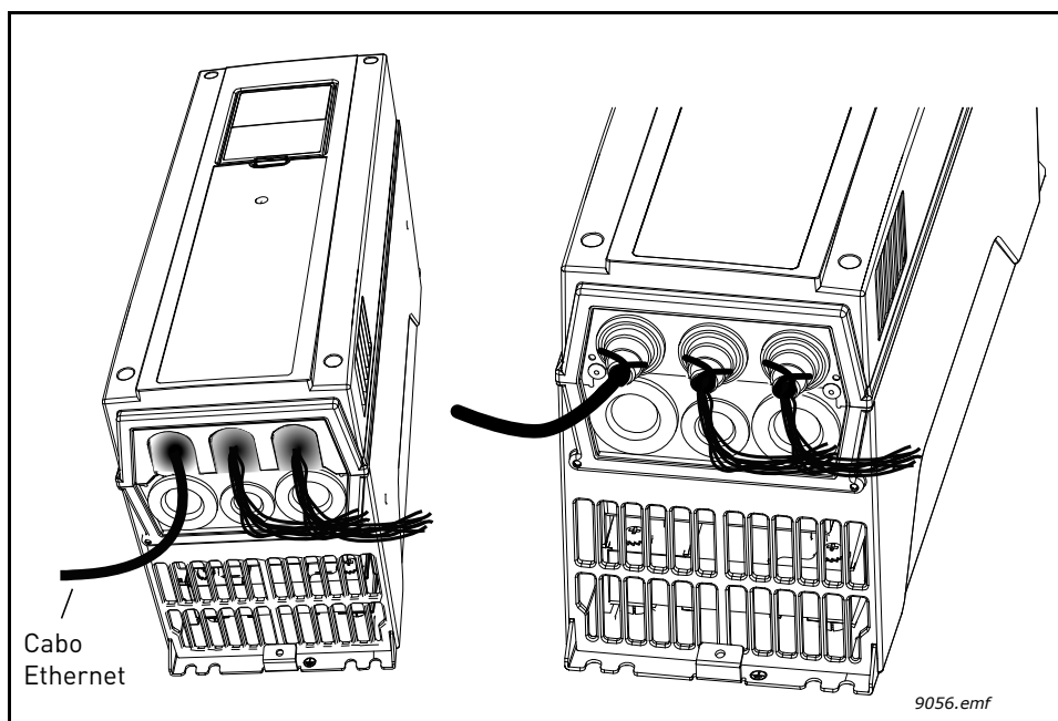
Figura 54. Distância entre cabos, esquerda: IP21, direita: IP54
