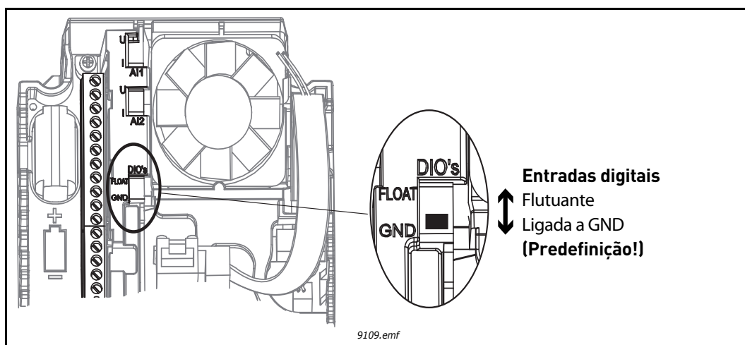
Figura 51. Altere a posição deste jumper para isolar as entradas digitais da terra.
