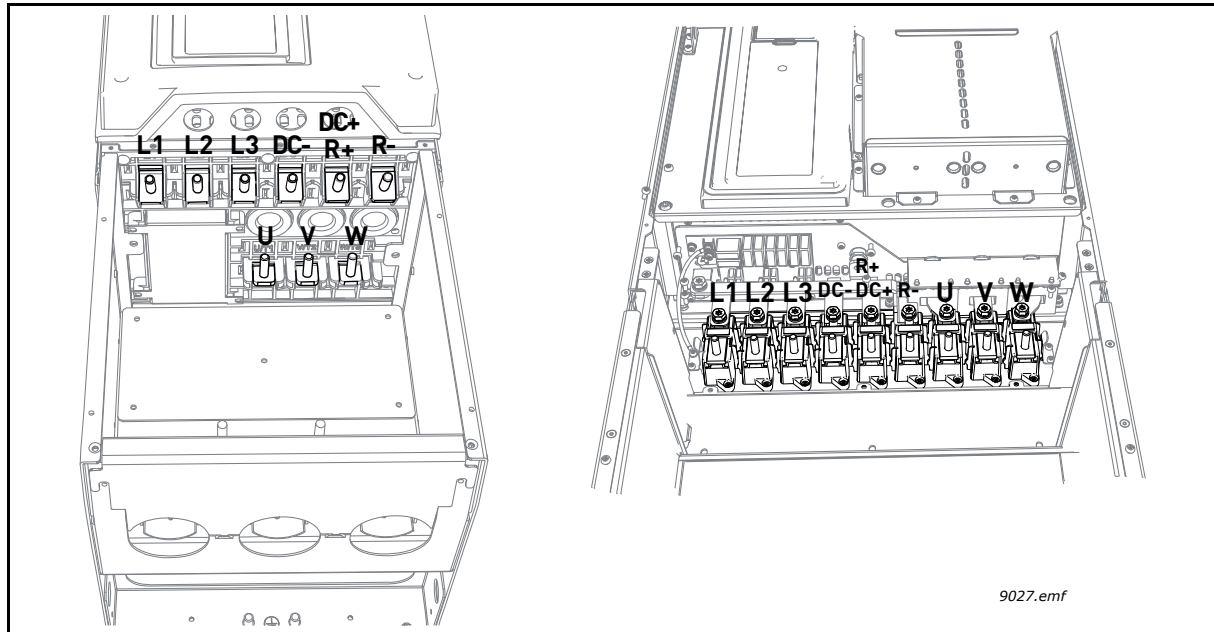
Figura 38. Terminais eléctricos, esquerda: MR8, direita: MR9
