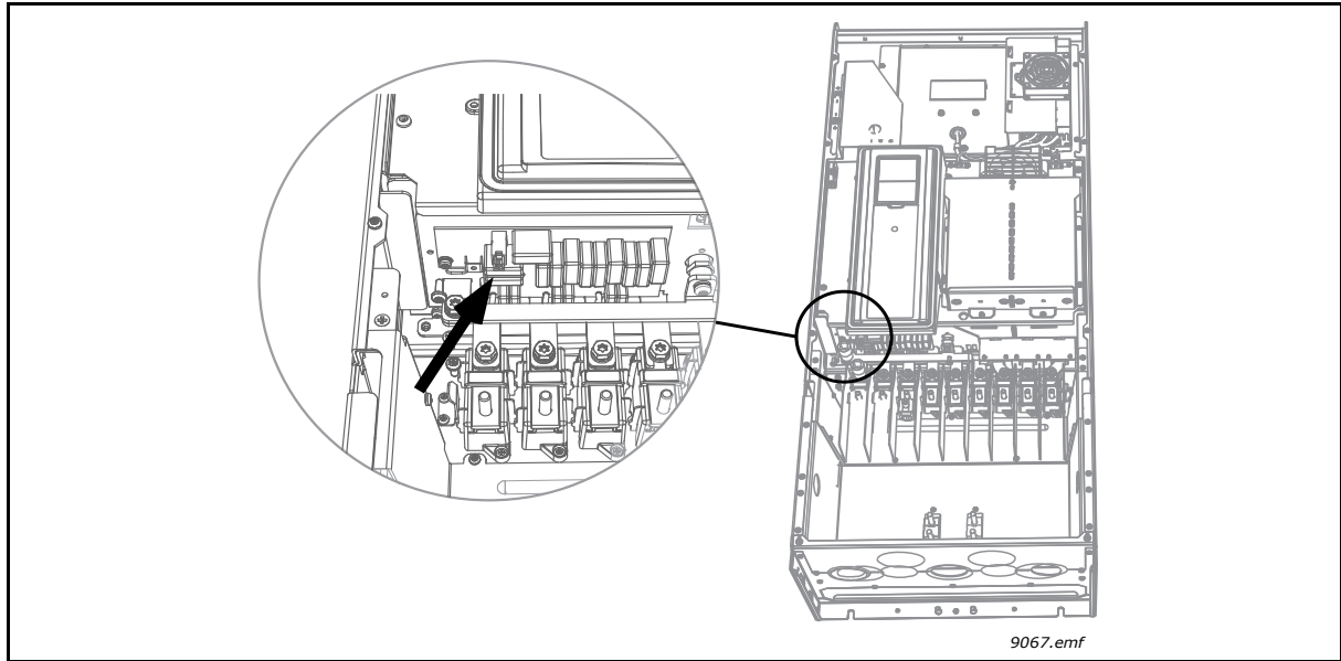
Figura 64. Retirar o jumper de EMC
