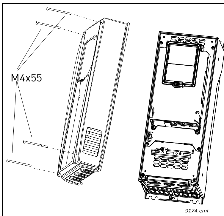
Figura 23. Abrir a tampa
