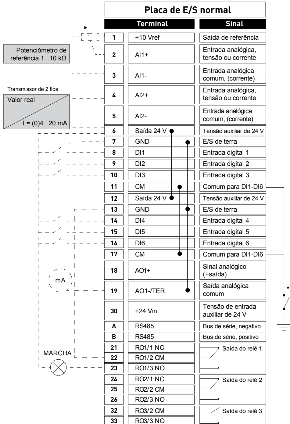
Figura 49. Sinais dos terminais de E/S de controlo na placa de E/S básica e exemplo de ligação
