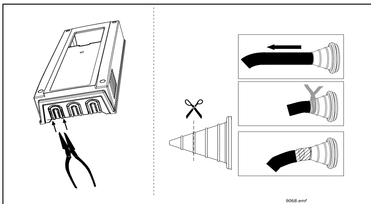
Figura 53. Conduzir os cabos, esquerda: IP21, direita: IP54
