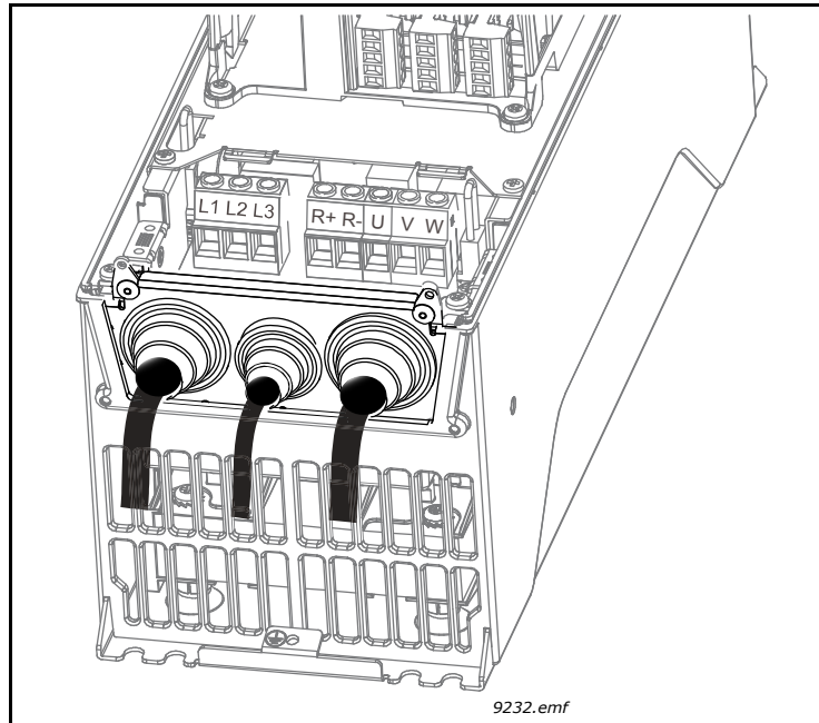
Figura 28. Placa passa-cabos e cabos
