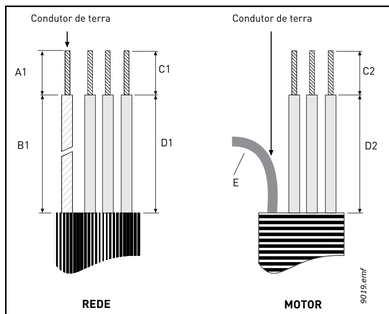
Figura 32. Descarnar os cabos
