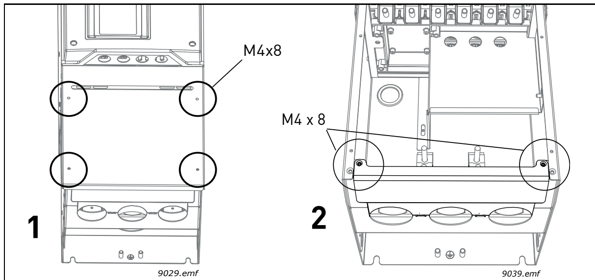
Figura 34. Retirar a tampa dos cabos e a placa de fixação dos cabos (MR8).
