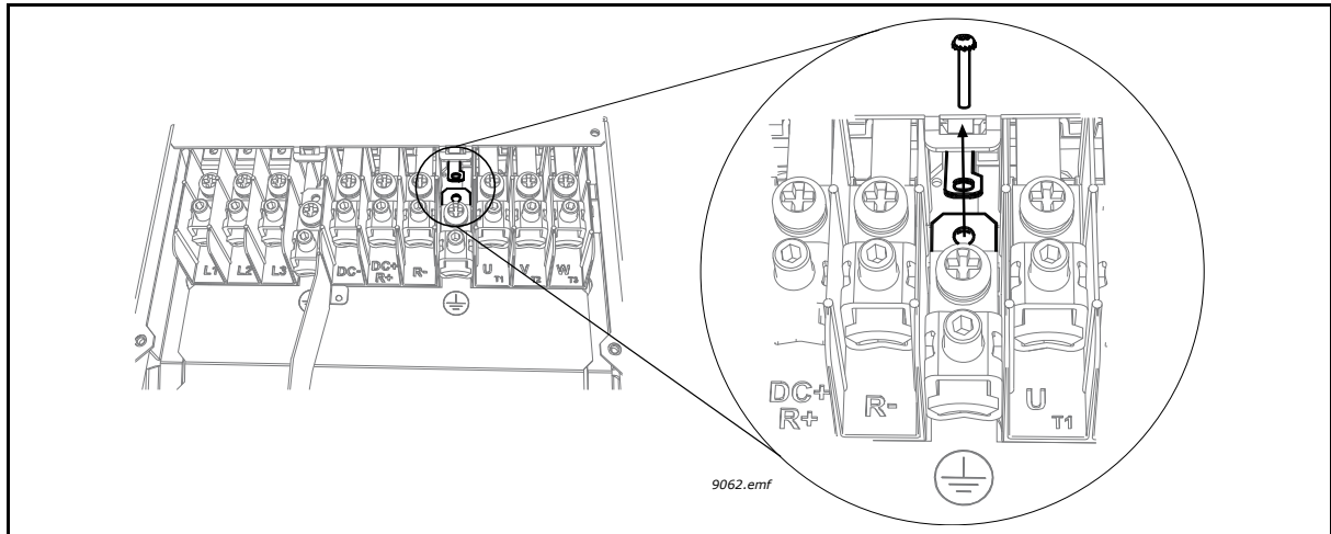
Figura 62. MR7: soltar o barramento de ligação à terra CC da estrutura
