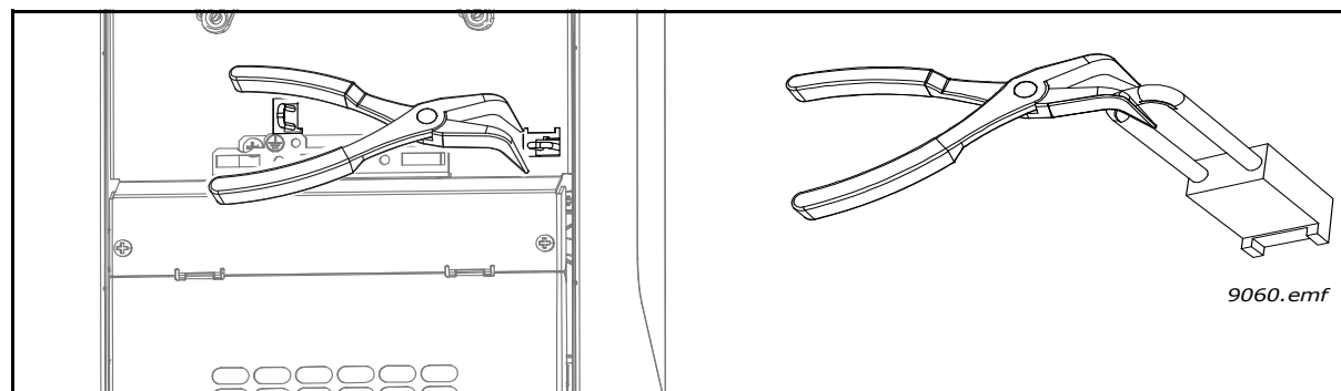
Figura 59. Retirar o jumper, MR6 como exemplo
