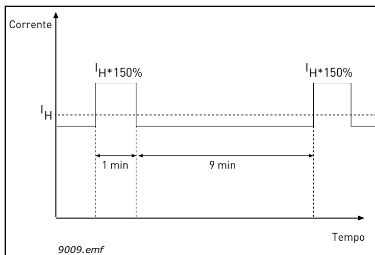
Figura 66. Alta sobrecarga
