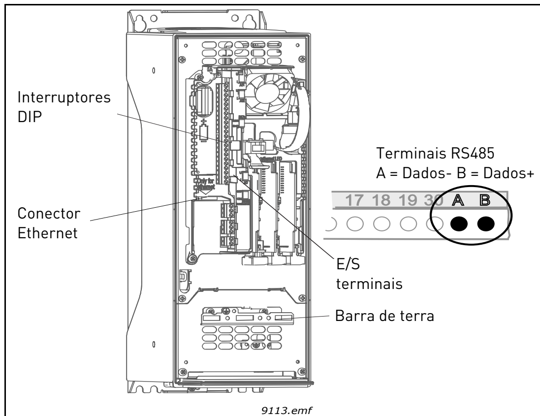
Figura 52. Ligações Ethernet e RS485
