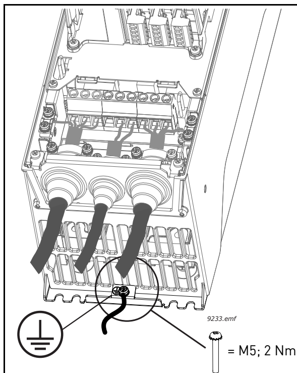
Figura 30. Conector adicional de ligação à terra de protecção
