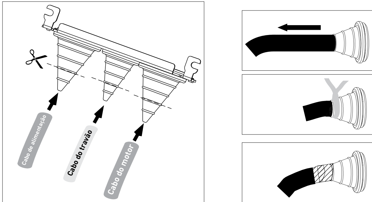
Figura 26. Corte e vedação dos anéis isolantes
