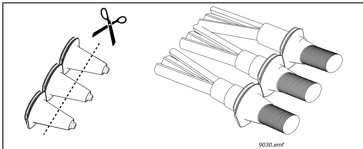
Figura 39. Cortar os anéis isolantes dos cabos
