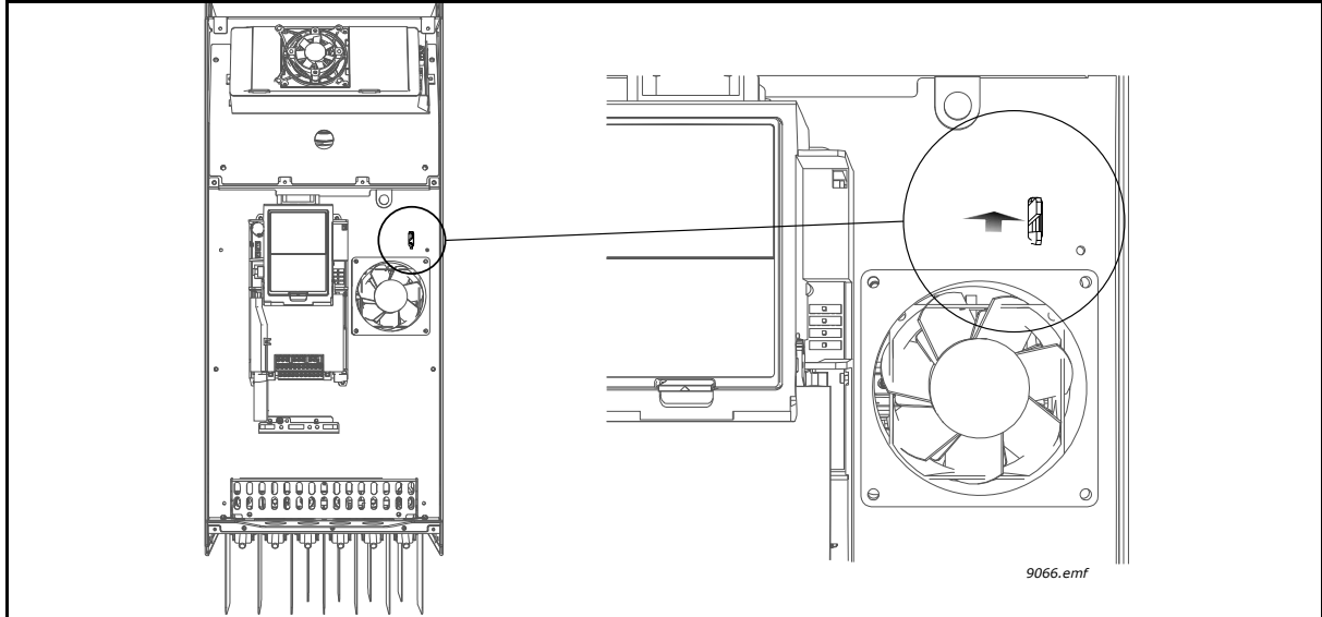
Figura 60. Braço de ligação à terra, MR8
