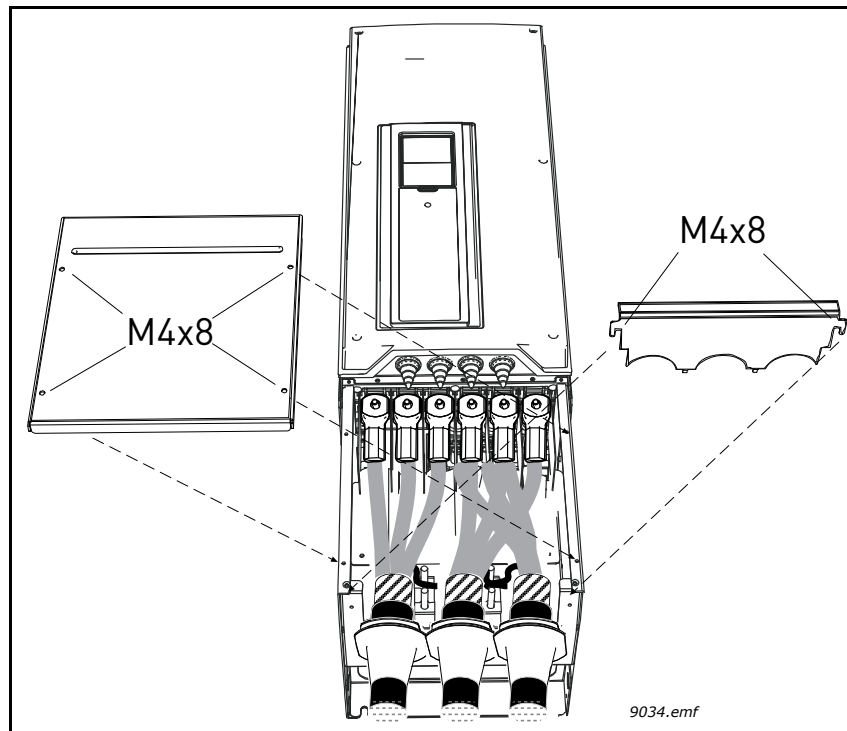
Figura 45. Recolocar a placa de fixação dos cabos e a tampa
