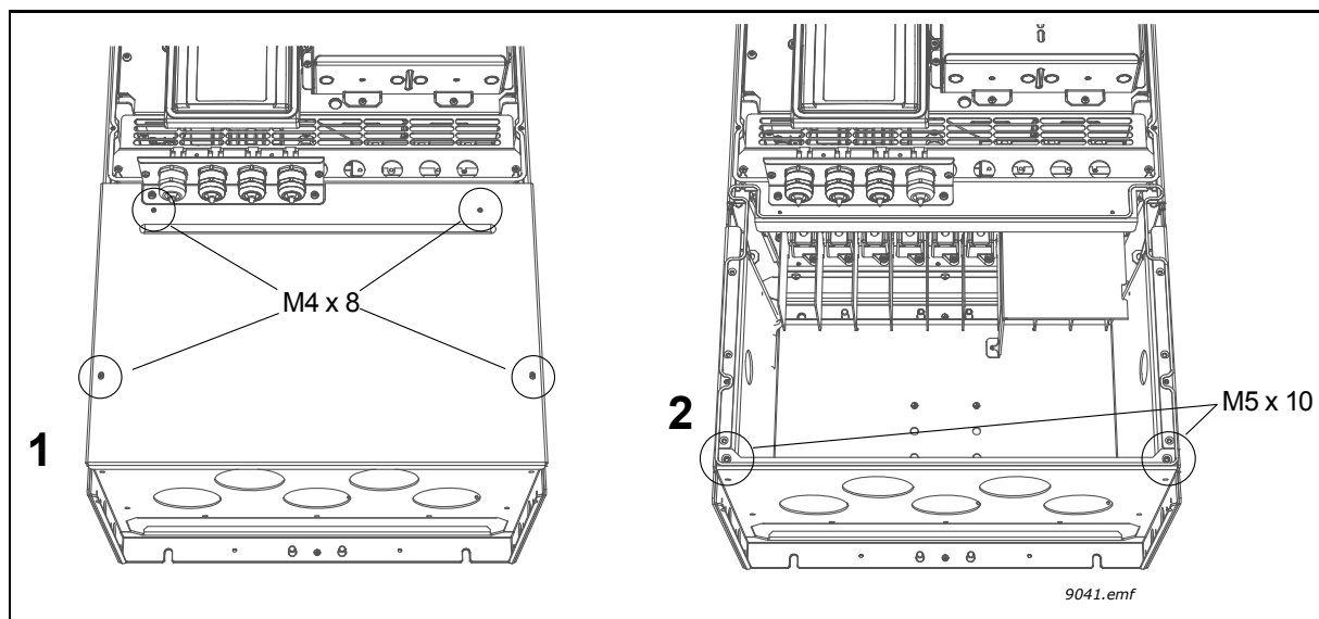
Figura 35. Retirar a tampa dos cabos e a placa de fixação dos cabos (MR9).
