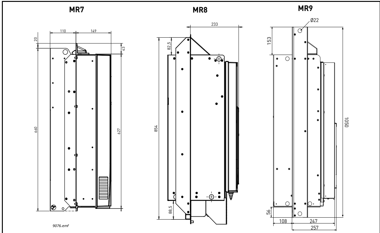
Figura 17. MR7 ao MR9, montagem com flange, dimensões de profundidade
