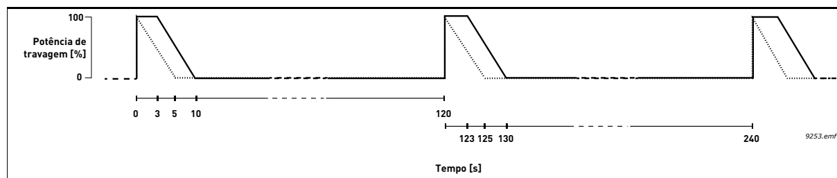
Figura 68. Ciclos de trabalho dos impulsos de PP e GP
