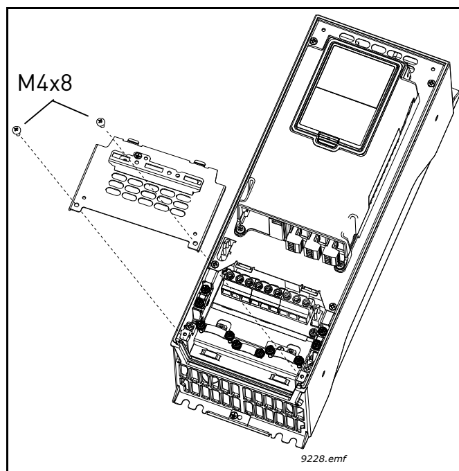
Figura 24. Retirar os parafusos
