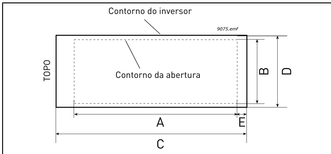
Figura 15. Dimensões do recorte para montagem com flange do MR7 ao MR9
