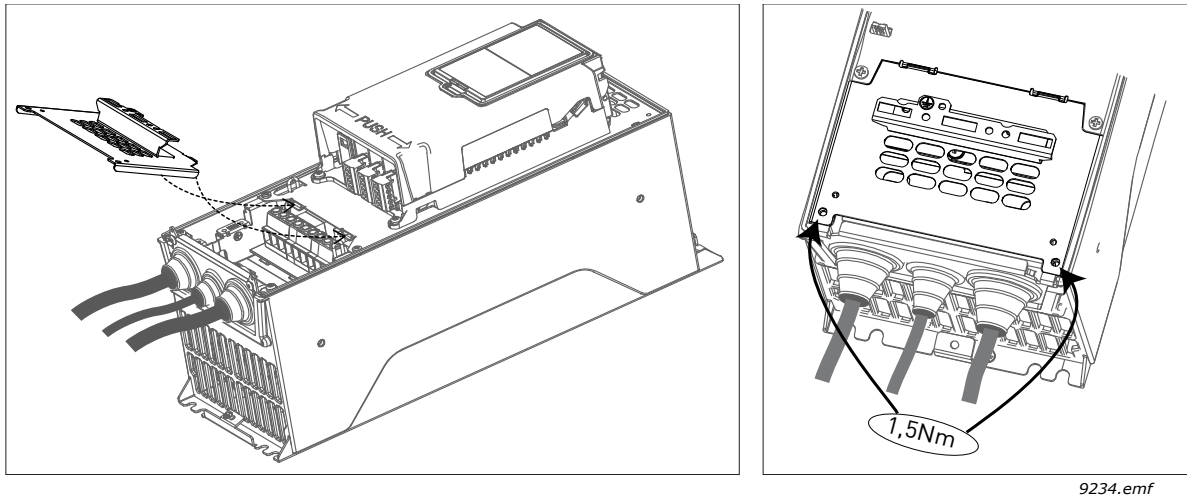
Figura 31. Reinstalar os componentes da tampa
