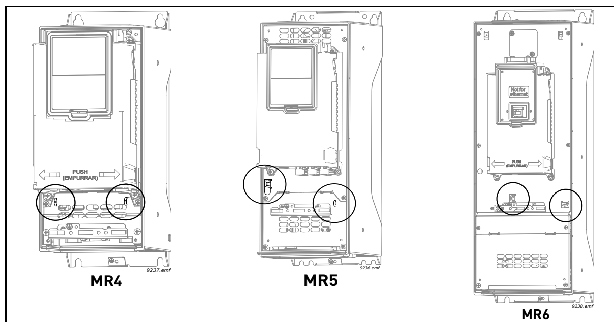
Figura 58. Localização dos jumpers de EMC nas estruturas MR4 a MR6
