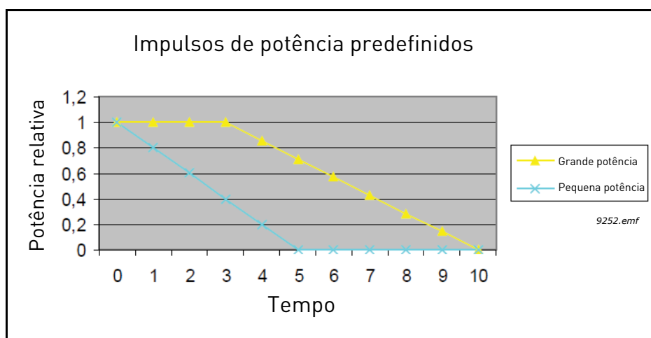
Figura 67. Formas dos impulsos de PP e GP
