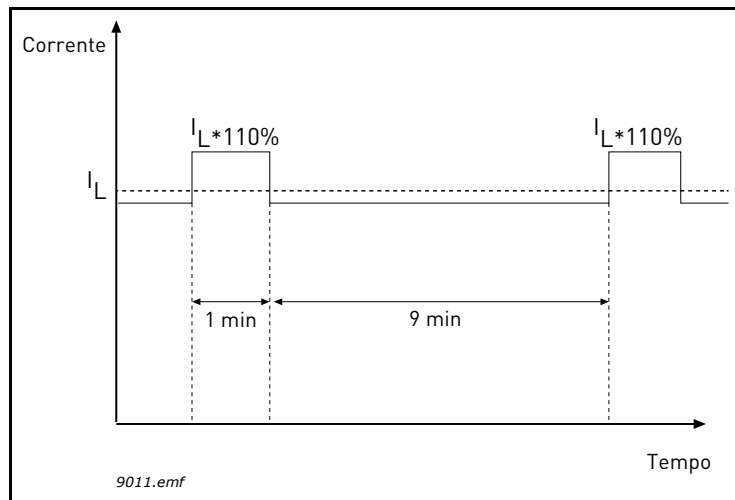
Figura 65. Baixa sobrecarga
