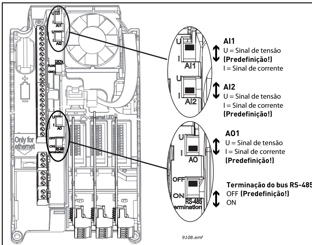
Figura 50. Interruptores DIP
