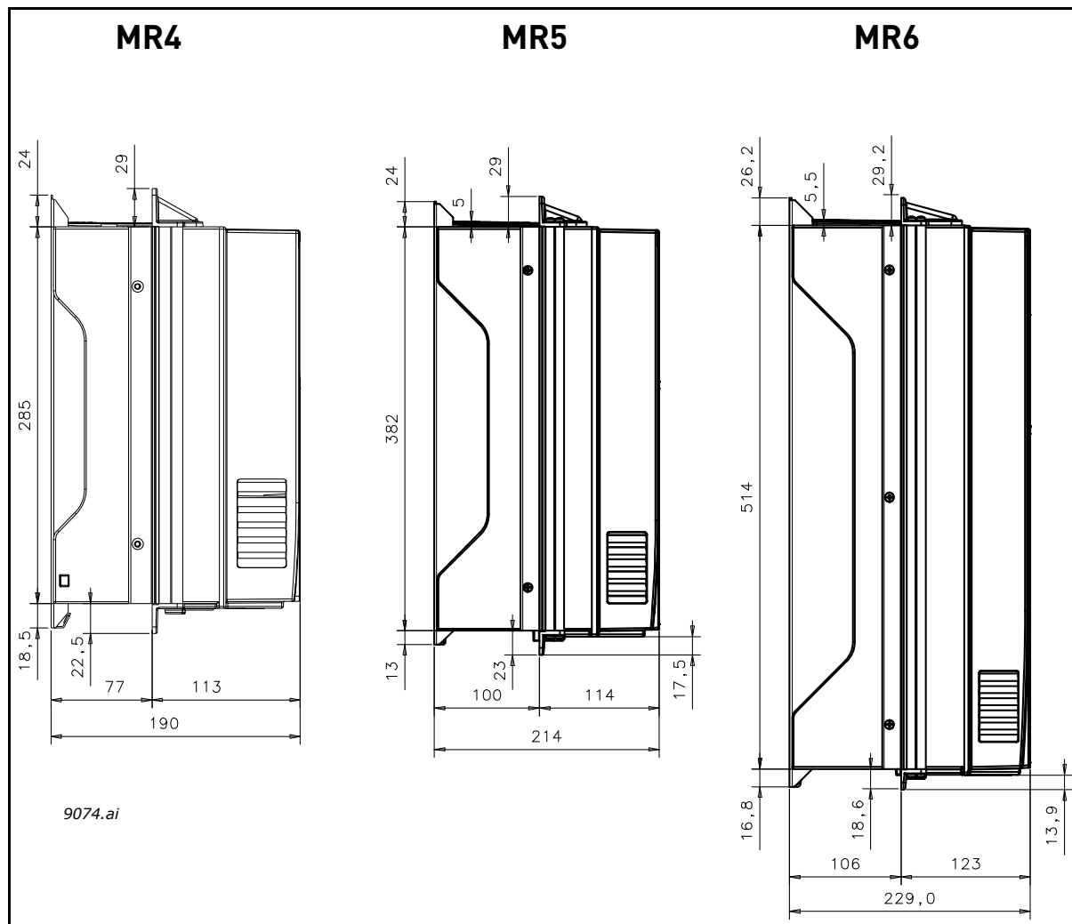
Figura 14. MR4 a MR6, montagem com flange, dimensões de profundidade
