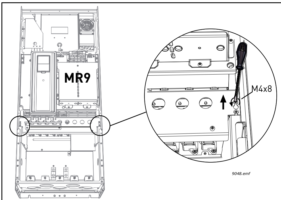
Figura 36. Retirar a placa de isolamento (MR9)
